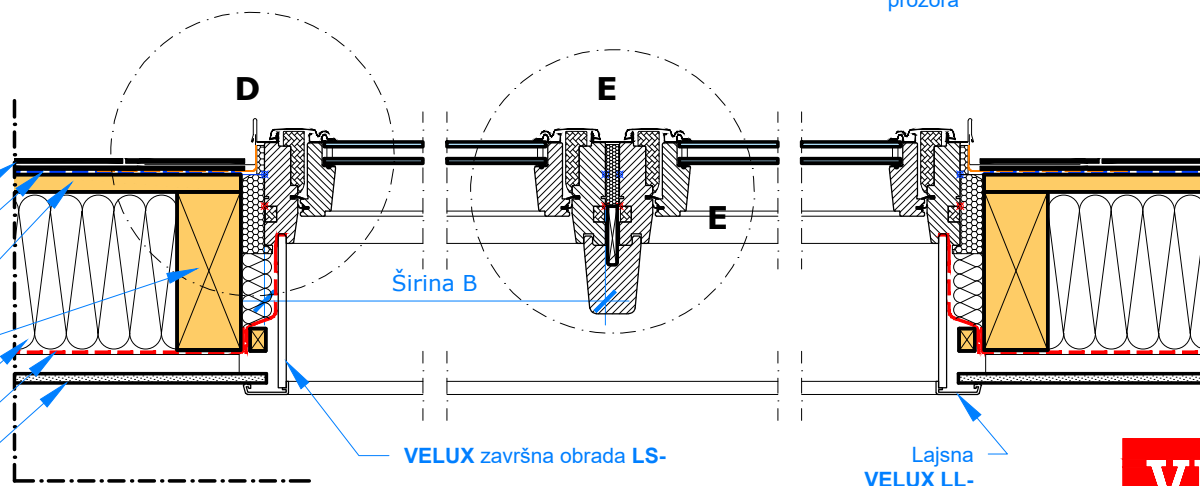
Odjeljak B-B / M10
